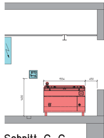
Schnitt C-C
