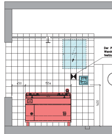
Schnitt B-B
