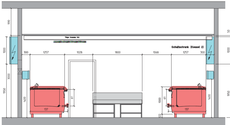
Schnitt A-A
