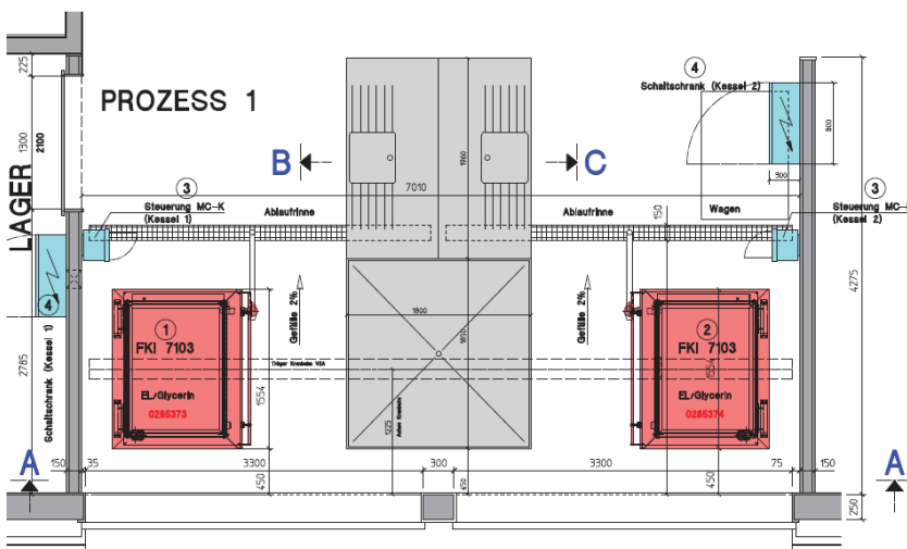
Draufsicht
